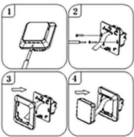
Obrázok 2. Demontáž termostatu
